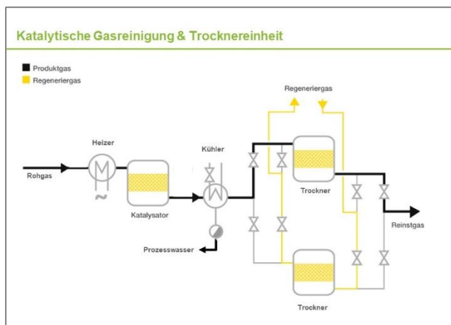
Vereinfachte Darstellung Sauerstoffreinigung
