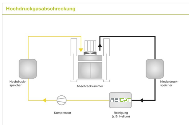
Anlagenschema
