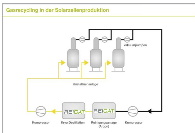
Anlagenschema
